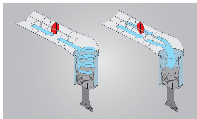
图 1: 涡流节气门: 沿着活塞轴向的涡流 左侧: 部分负荷, 涡流节气门闭合, 强涡流 右侧: 全负荷, 涡流节气门开启, 进气程度高
